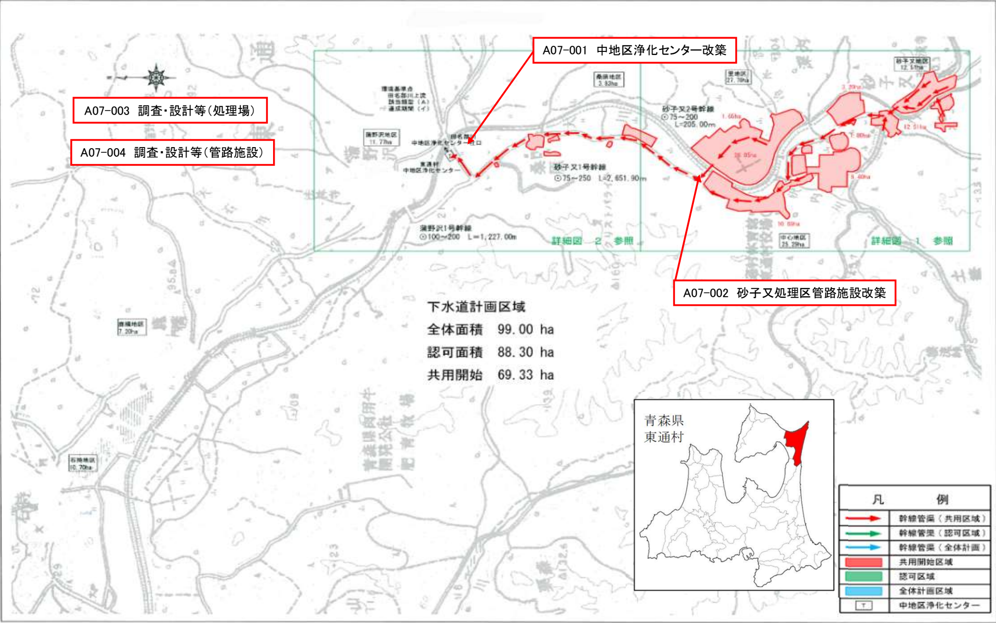
東通村特定環境保全公共下水道 全体図
