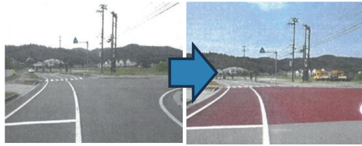
東通小学校前の交差点のカラー舗装
